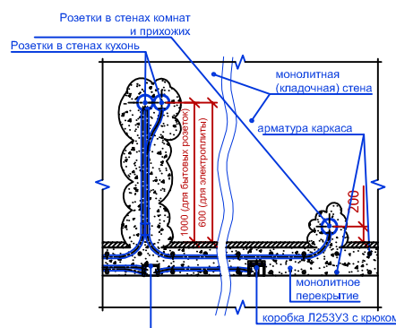
Эскиз 1. Монтаж полипропиленовых труб (ПП), распаячных и установочных коробок в монолите перекрытия (пола) и в стенах.
